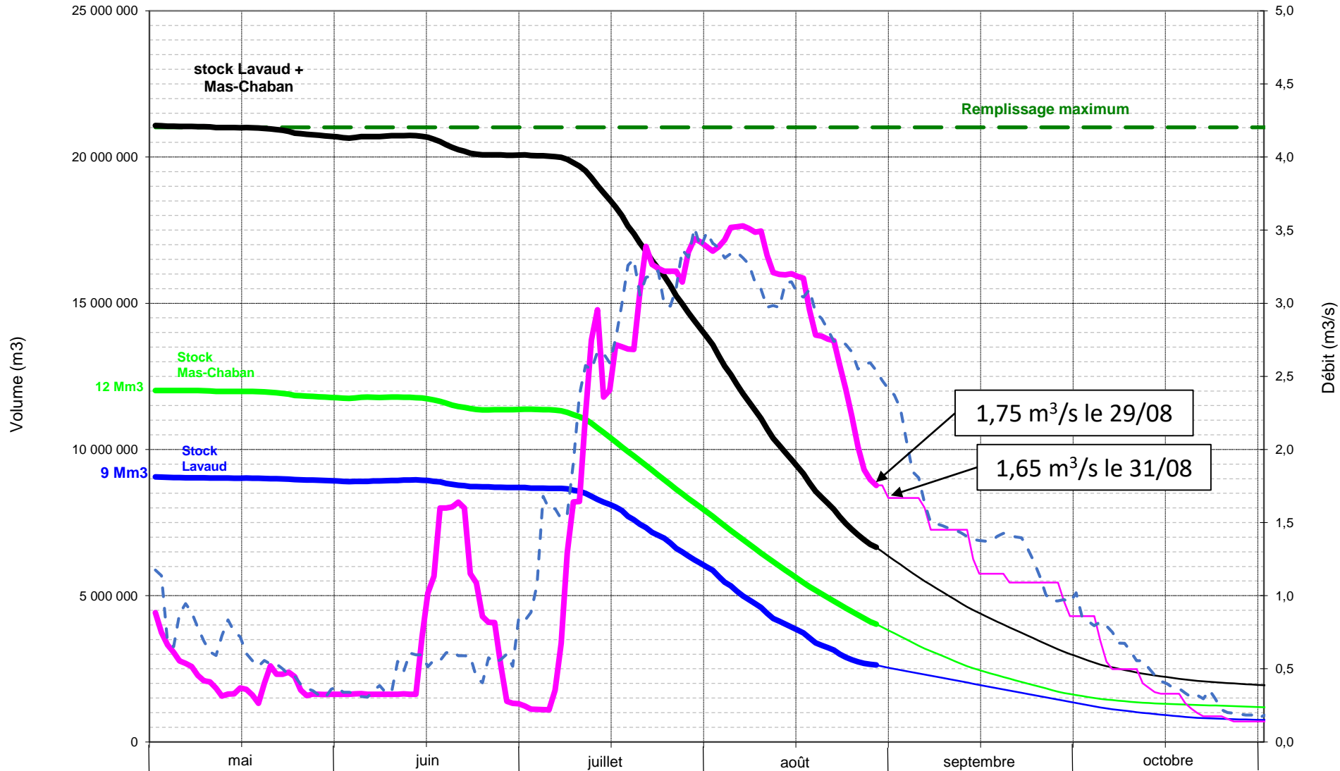
Scénario de lâchures des barrages de Lavaud et Mas-Chaban - Etiage 2022
