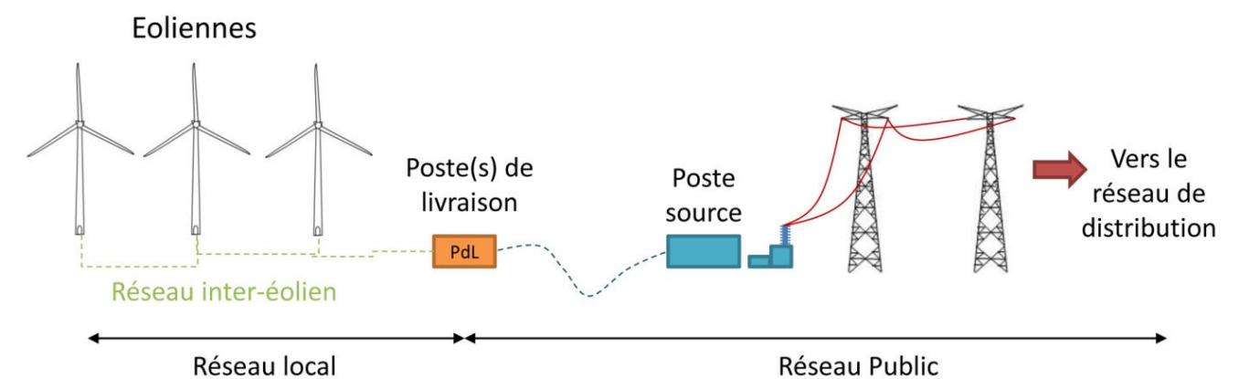
Figure 6 : Raccordement électrique des installations (Source : Guide technique, mai 2012)
