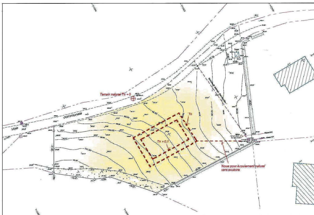
Figure 3 Prévision d'une noe d'évacuation des eaux sur le plan masse du permis de construire
