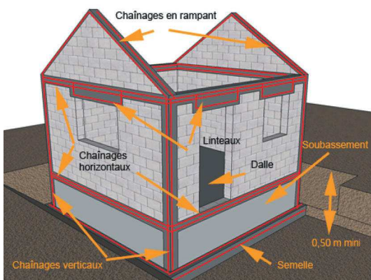
Figure 30 Schéma de principe des chaînages de maison individuelle (Source abc maçonnerie.com)
