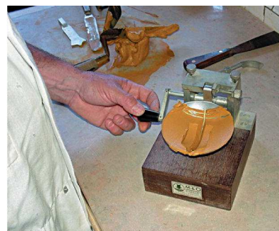
Figure 9 Détermination de la limite de plasticité au cône (à gauche) et à la coupelle de Casagrande (à droite) (Source Cerema)
