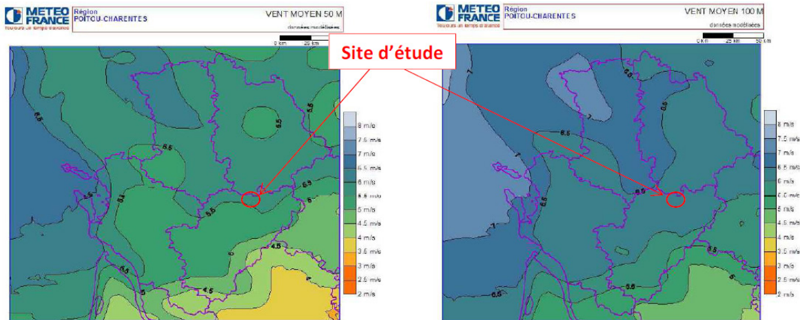
Vitesse moyenne du vent à une hauteur de 50 m
