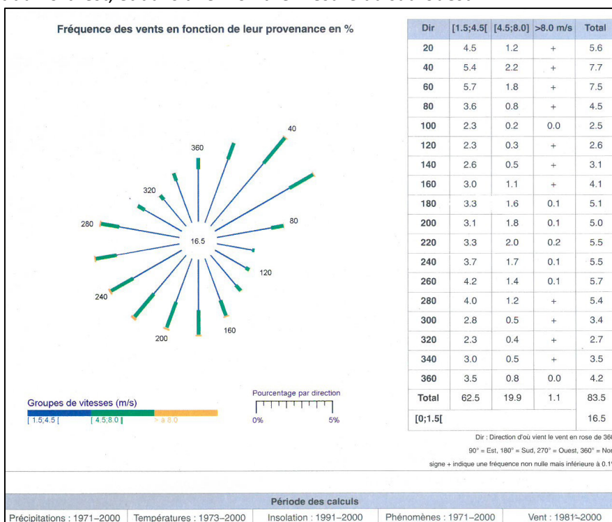
Figure 13 : Rose des vents - Station de Limoges (Source : Météo France)
