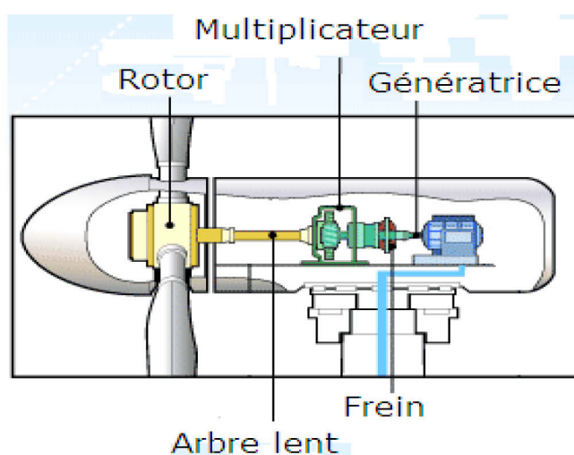
Figure 7: Schéma simplifié de la chaîne cinématique
