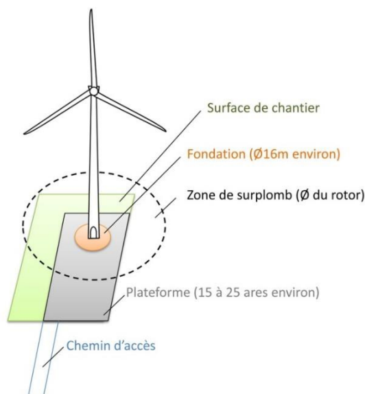
Figure 4 : Illustration des emprises au sol d'une éolienne
