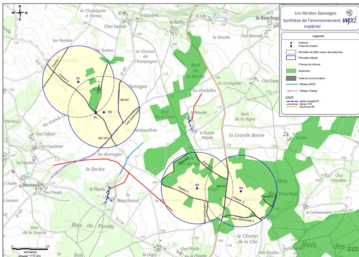
Figure 19 : Synthèse de l'environnement matériel du projet éolien des Herbes Sauvages
