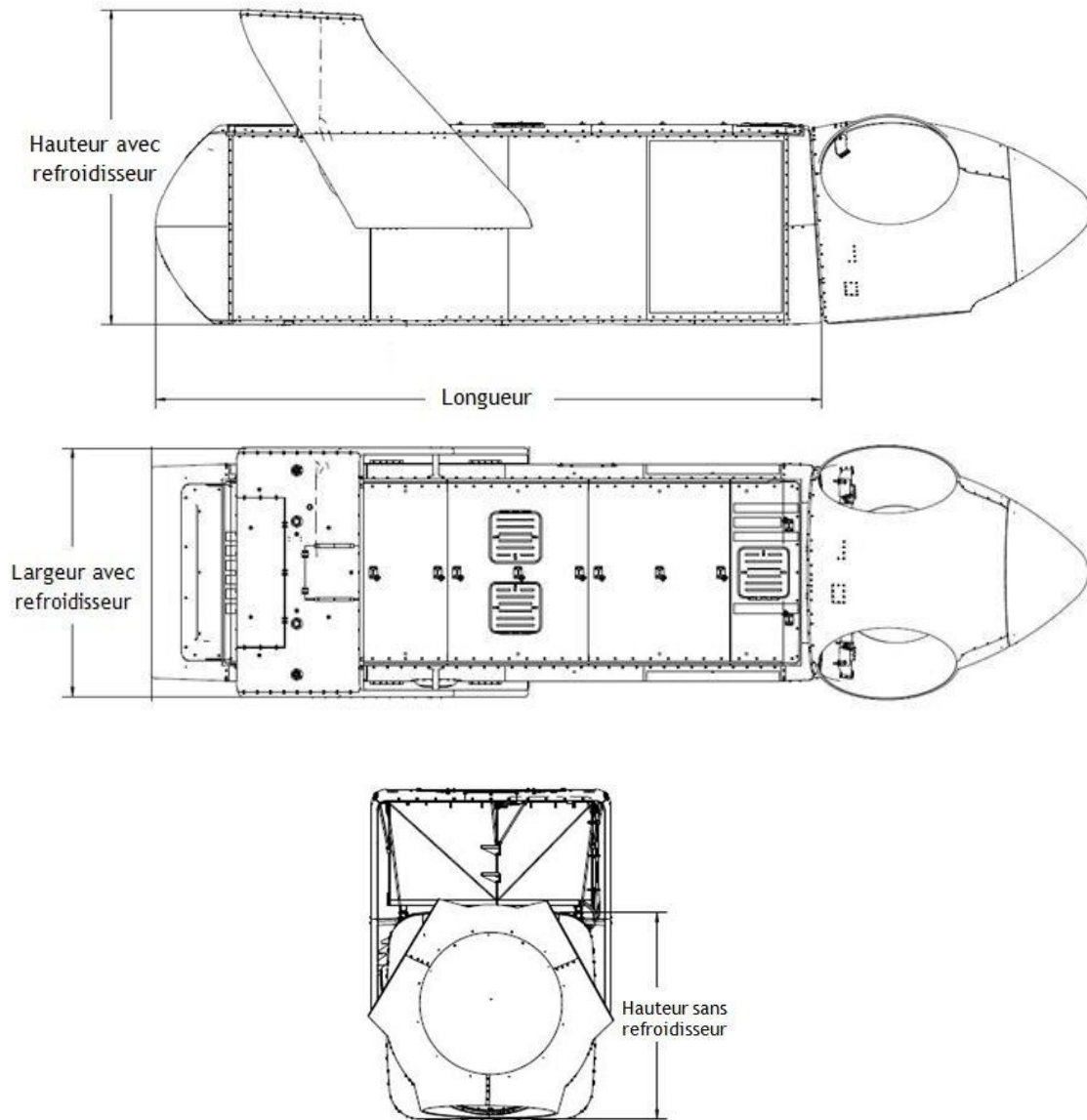
Figure 6: dimensions d'une nacelle
