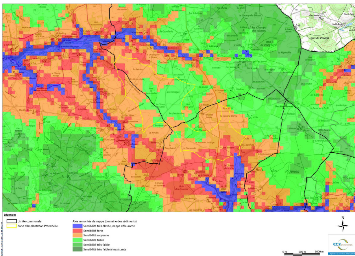
Figure 16: Risque de remontée de nappe au niveau de la zone d'implantation potentielle du projet (domaine des sédiments)
