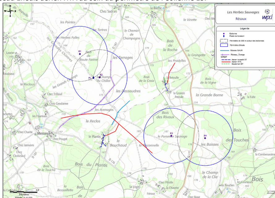
Figure 18 : Réseaux et servitudes au niveau de la zone d'implantation du projet éolien des Herbes Sauvages
