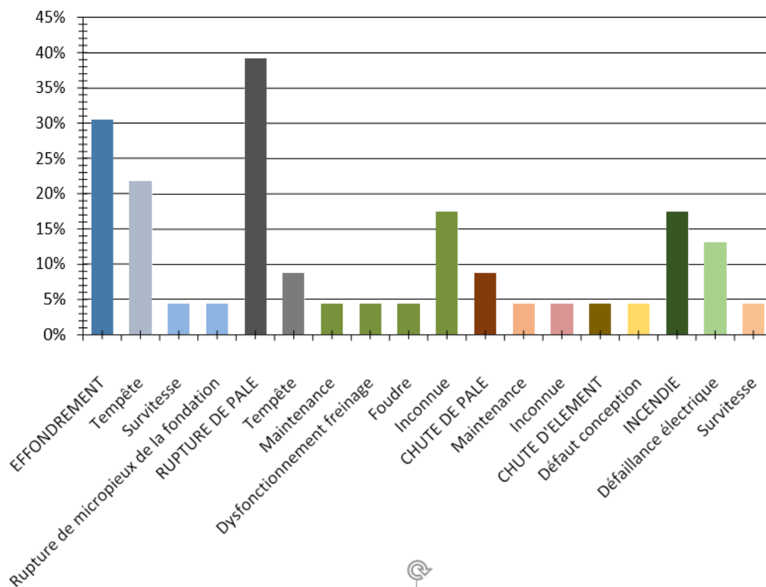
Figure 20 : Répartition des événements accidentels et de leurs causes premières sur le parc d'aérogénérateur français entre 2000 et 2011
