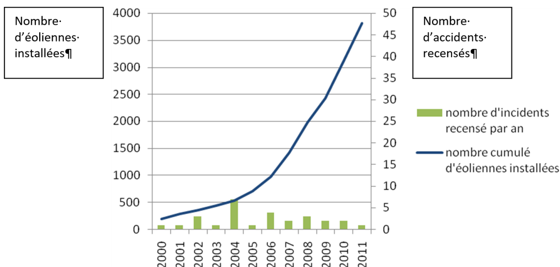
Figure 24 : Evolution du nombre d'incidents annuels en France et nombre d'éoliennes installées
