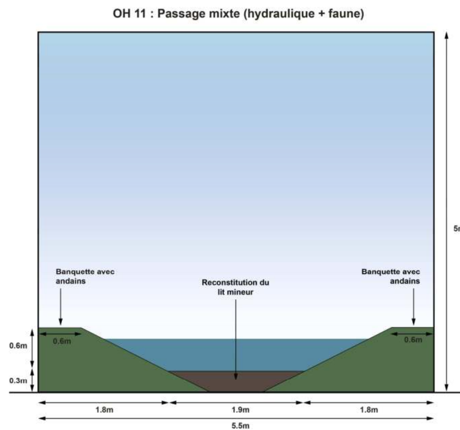
FIGURE 6 : COUPE DE PRINCIPE POUR OUVRAGE DE FRANCHISSEMENT OH11
