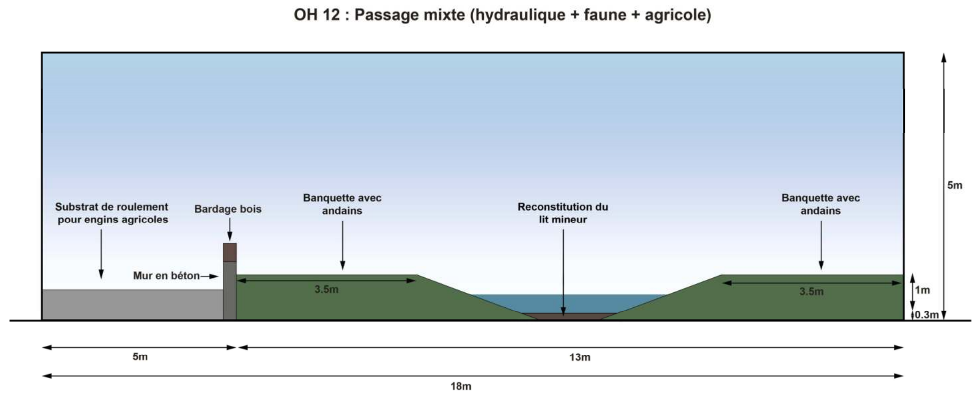
FIGURE 7 : COUPE DE PRINCIPE POUR OUVRAGE DE FRANCHISSEMENT OH12
