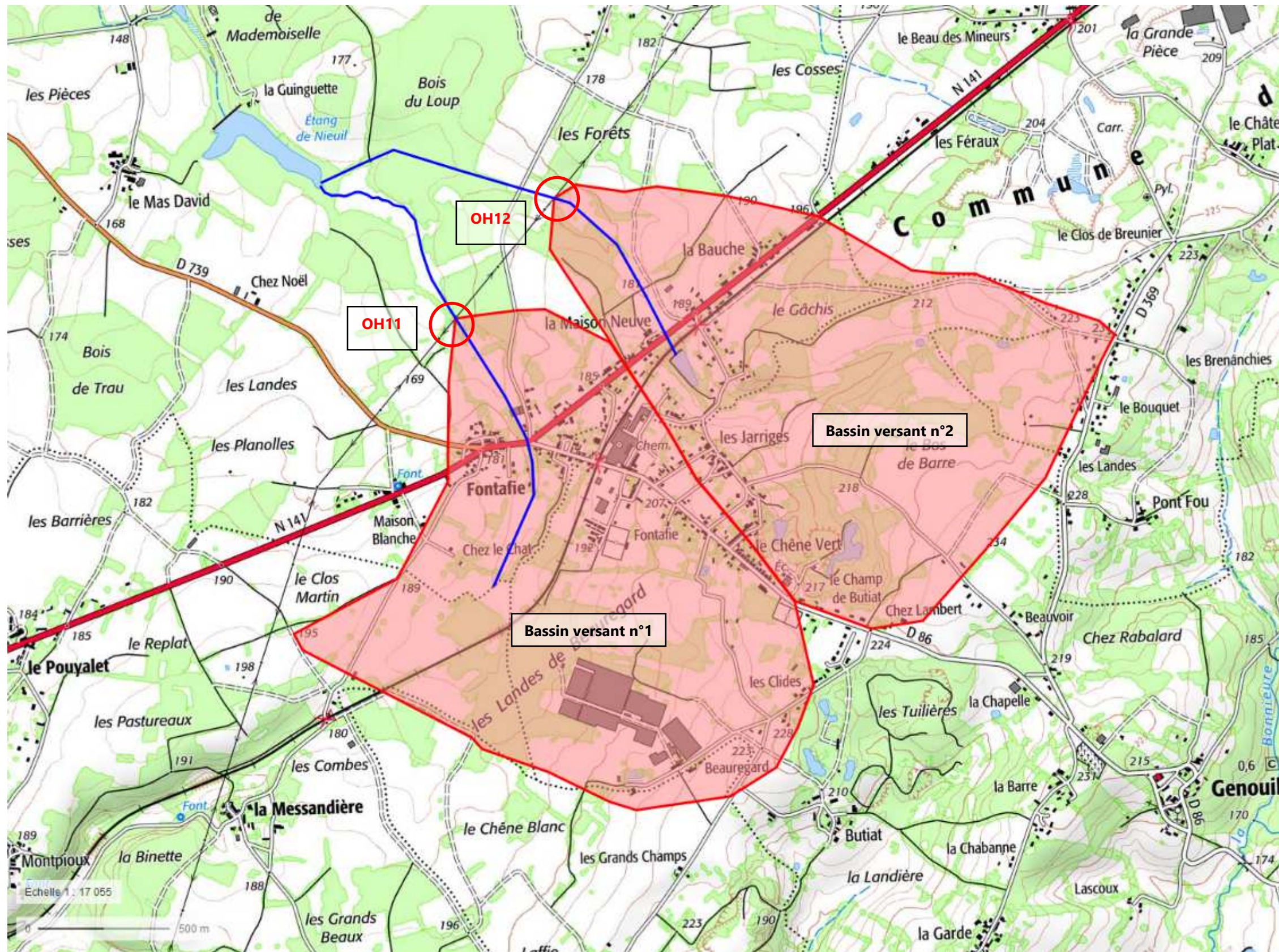
FIGURE 8 : PLAN DES BASSINS VERSANTS DES DEUX COURS D'EAU IMPACTES PAR LA MISE A DEUX FOIS DEUX VOIES DE LA RN141
