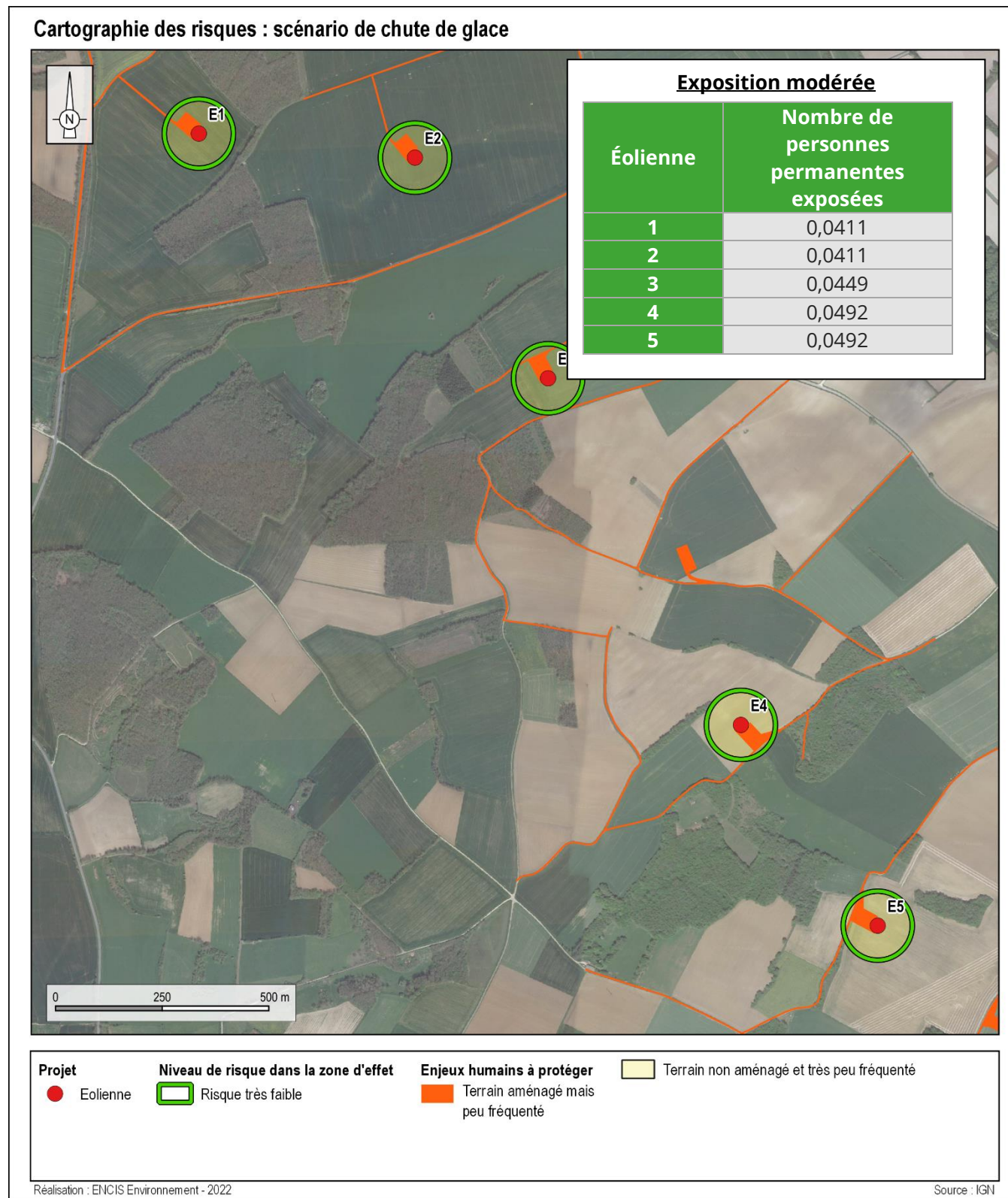
Carte 7 : Cartographie des risques – Scénario de chute de glace
