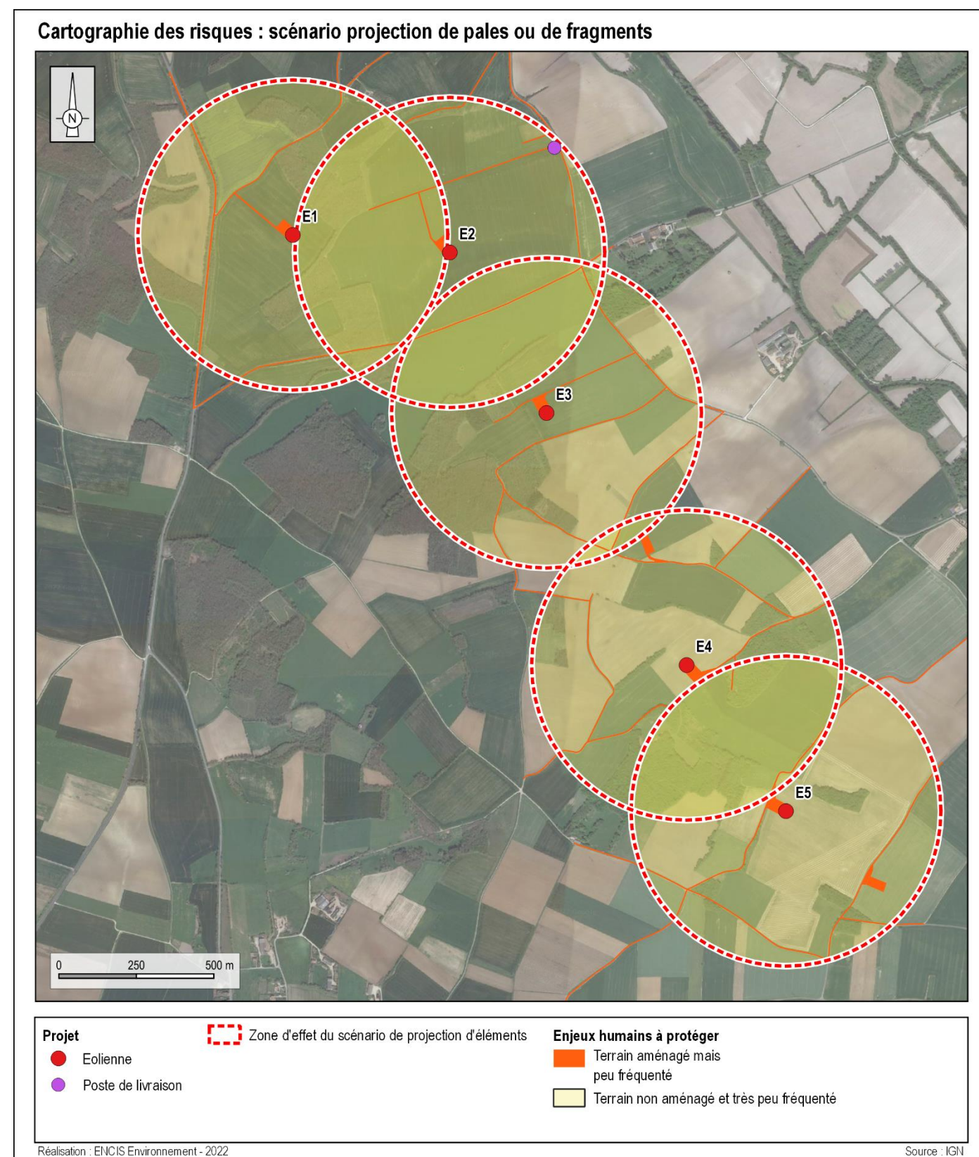
Carte 16 : Cartographie des enjeux identifiés dans les zones d'effet du scénario de projection de pales ou de fragments de pales
