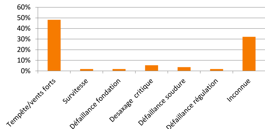
Figure 8 : Répartition des causes premières d'effondrement dans les accidents à l'international entre 2000 et 2011 (Source : Guide technique, mai 2012)
