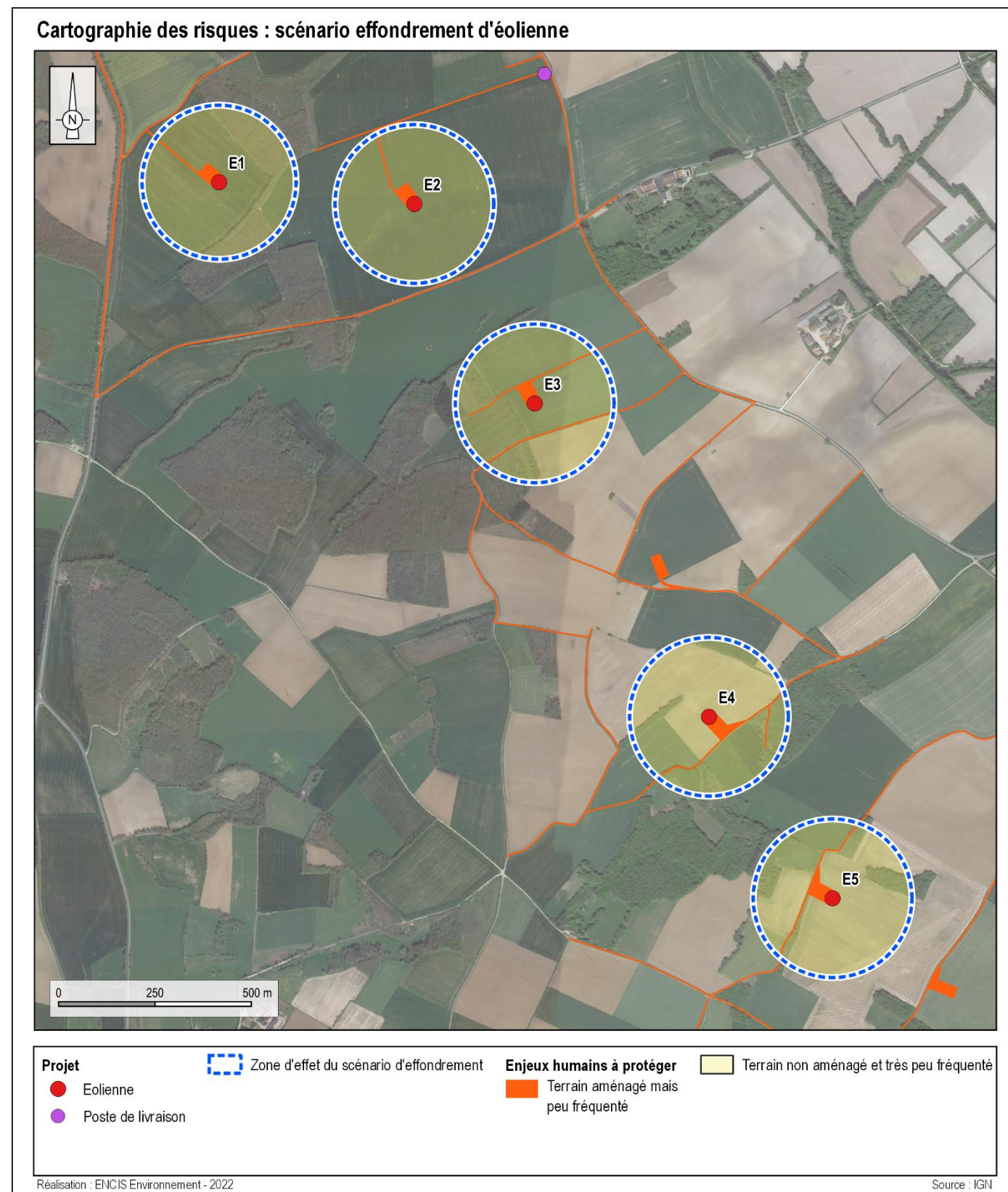
Carte 13 : Cartographie des enjeux identifiés dans les zones d'effet du scénario d'effondrement d'éolienne
