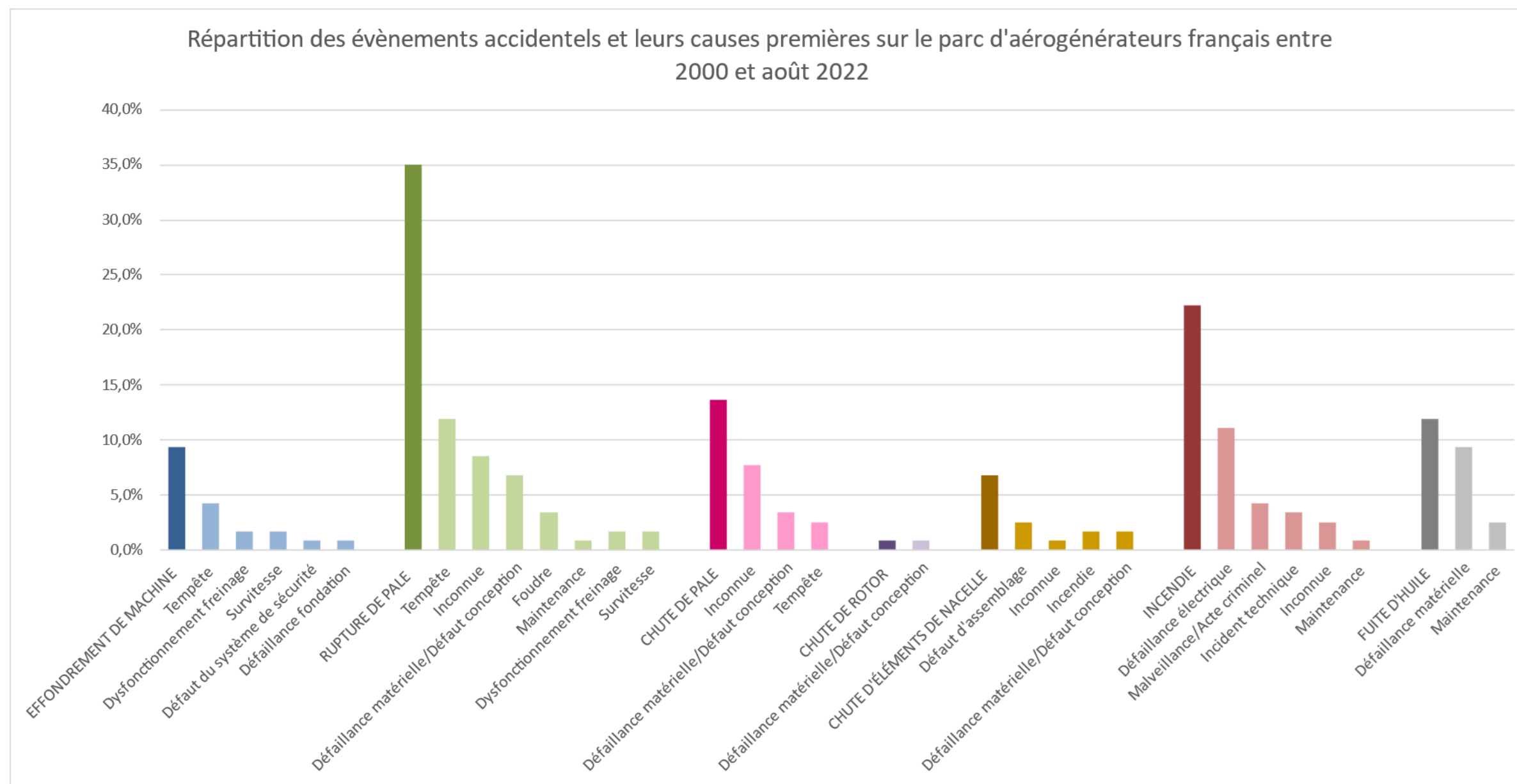
Figure 6 : Répartition des accidents et de leurs causes premières sur le parc éolien français entre 2000 et août 2022
