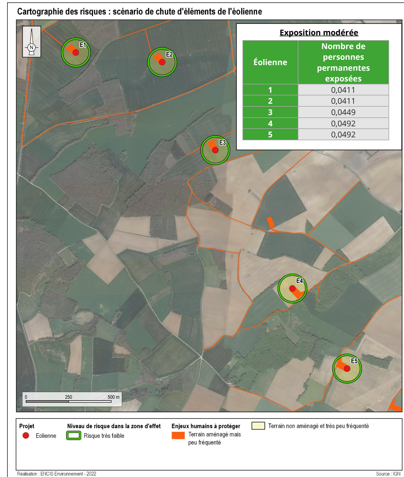
Carte 8 : Cartographie des risques – Scénario de chute d'éléments de l'éolienne
