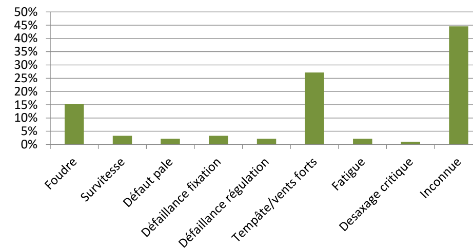
Figure 9 : Répartition des causes premières de rupture de pale dans les accidents à l'international entre 2000 et 2011 (Source : Guide technique, mai 2012)
