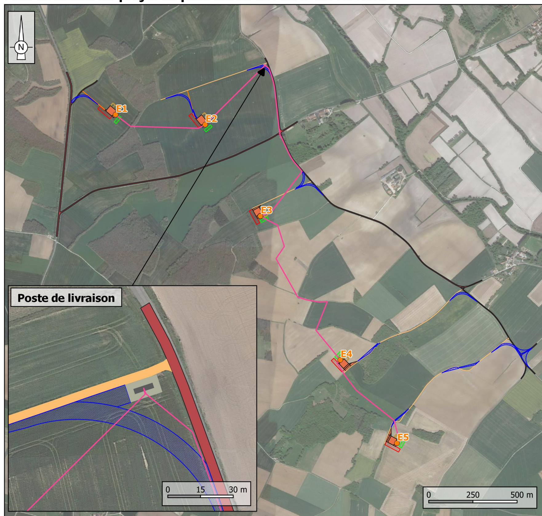
Carte 5 : Plan du projet de parc éolien de Marcillac-Lanville
