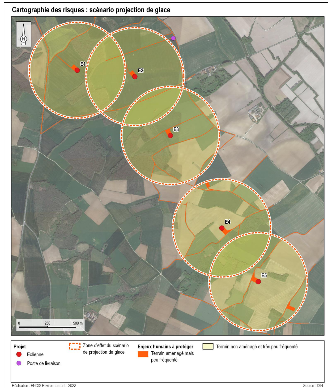
Carte 17 : Cartographie des enjeux identifiés dans les zones d'effet du scénario de projection de glace
